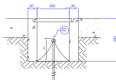
CORTE A-A (S/ ESCALA)
