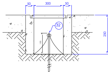
DETALHE 1 ATERRAMENTO (S/ ESCALA)
