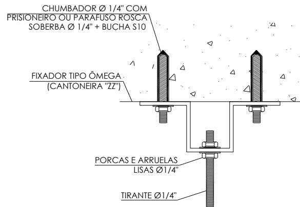
DETALHE 1 (S/ESCALA)
