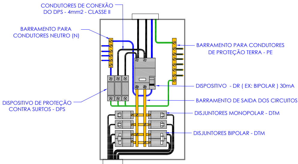
DETALHE 1
