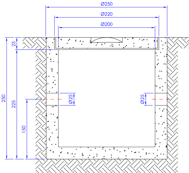
Corte AA
