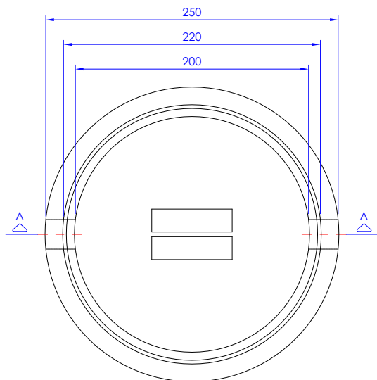
Vista superior
